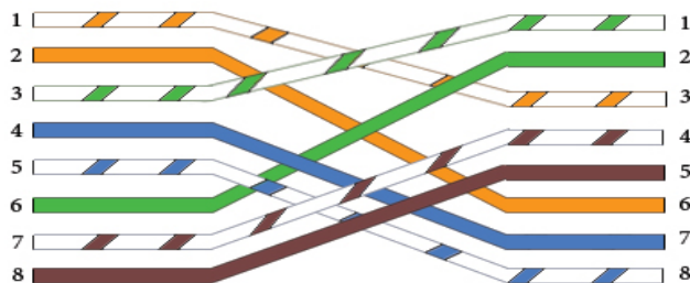
Crossover Wiring Guide 568-B
